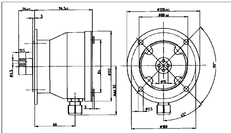
Fig. 2: Dimensions
